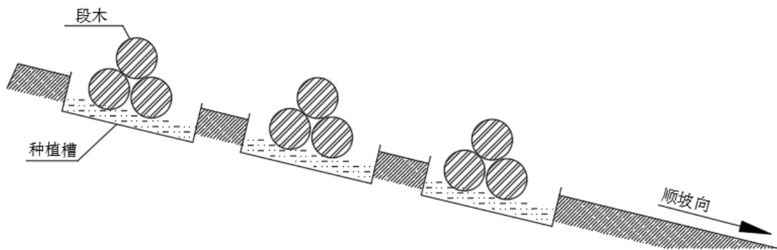
图4 段木摆放纵截面示意图
