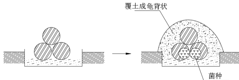
图6 菌种贴放示意图
