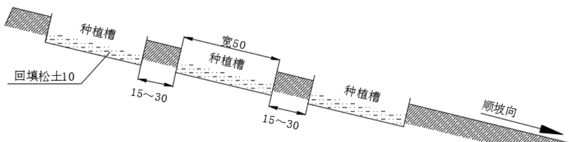
图2 种植槽纵截面示意图
