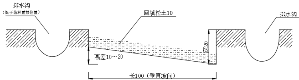
图1 种植槽横截面示意图
